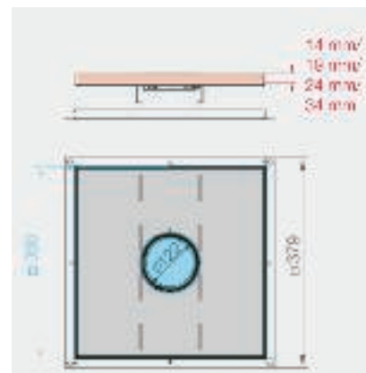
RKFSL, tubusos 250-3 névleges méret, 2. terhelési osztály
