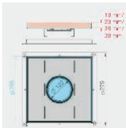
RKFSL, tubusos 250-3 névleges méret, 1. terhelési osztály
